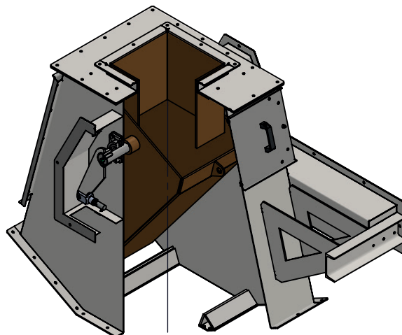
Distributeur pendulaire pneumatique 1 entrée / 3 sorties
