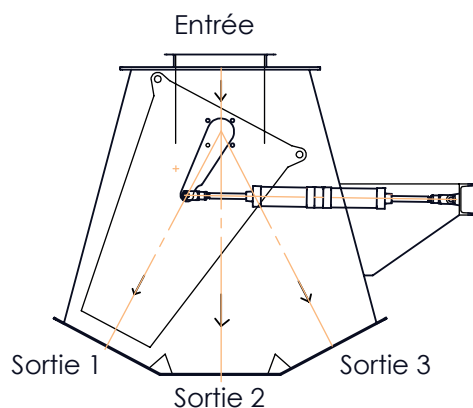
Distributeur pendulaire pneumatique 1 entrée / 3 sorties
