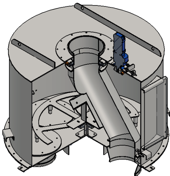
Distributeur simple entrée
