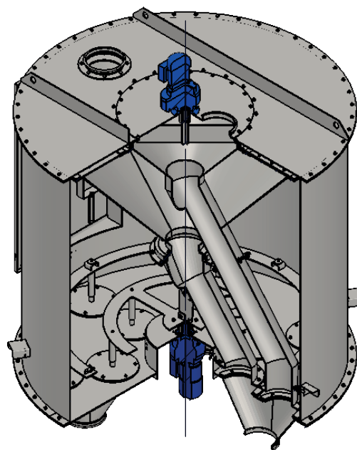
Distributeur double entrées
