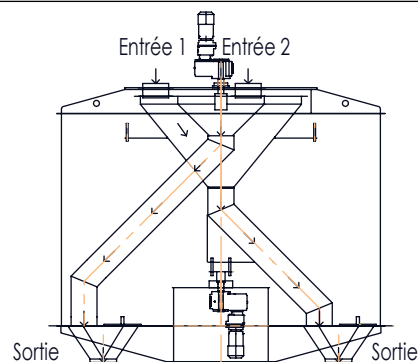
Distributeur double entrées
