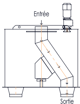
Distributeur simple entrée
