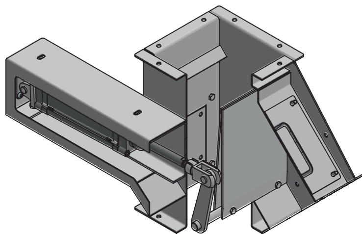
B2D 45° asymétrique
